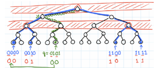
INTEGERS
